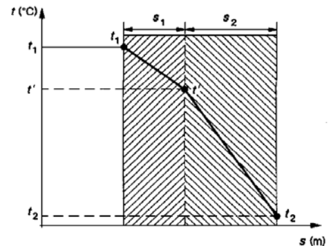
Figura 2. Parete composta
