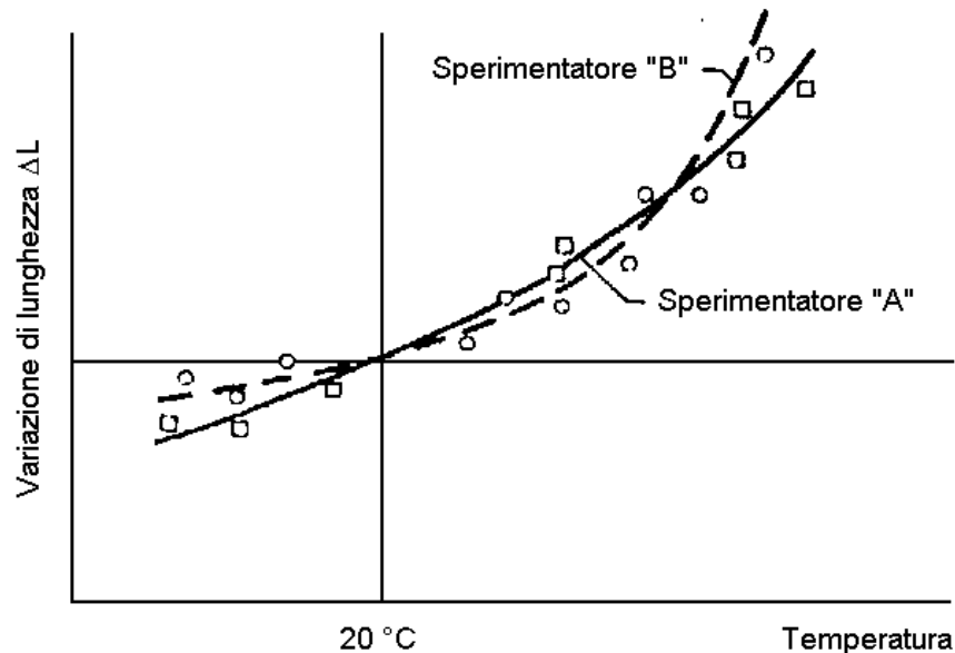
Figura 6. Misure di dilatazione termica
